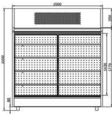
• نمای روبروی یخچال صدف پرده هوا (موتور بالا)
