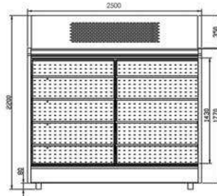
• نمای روبروی یخچال صدف پرده هوا (موتور بالا)
