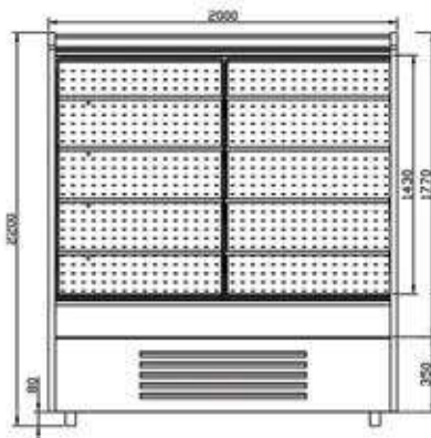
• نمای روبروی یخچال صدف پرده هوا (موتور پایین)
