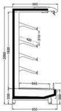
طبقات بصورت شیب دار
