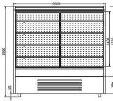
• نمای روبروی یخچال صدف پرده هوا (موتور پایین)
