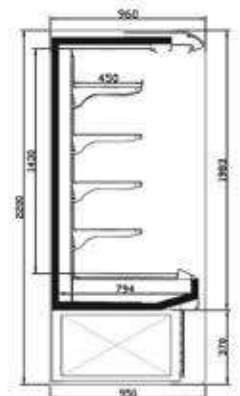
• نمای مجاور (موتور پایین)
