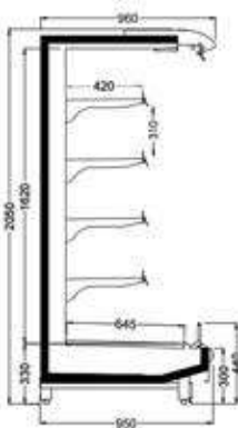
طبقات بدون شیب
