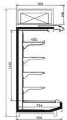
• نمای مجاور (موتور بالا)
