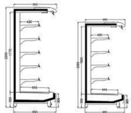
نمای مجاور کریستال (Height 2050/2200)
